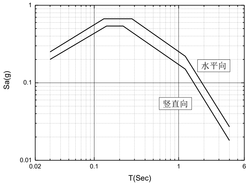
附图 1 场址 SL-2 级设计基准地面运动基岩加速度反应谱（5%阻尼比）
